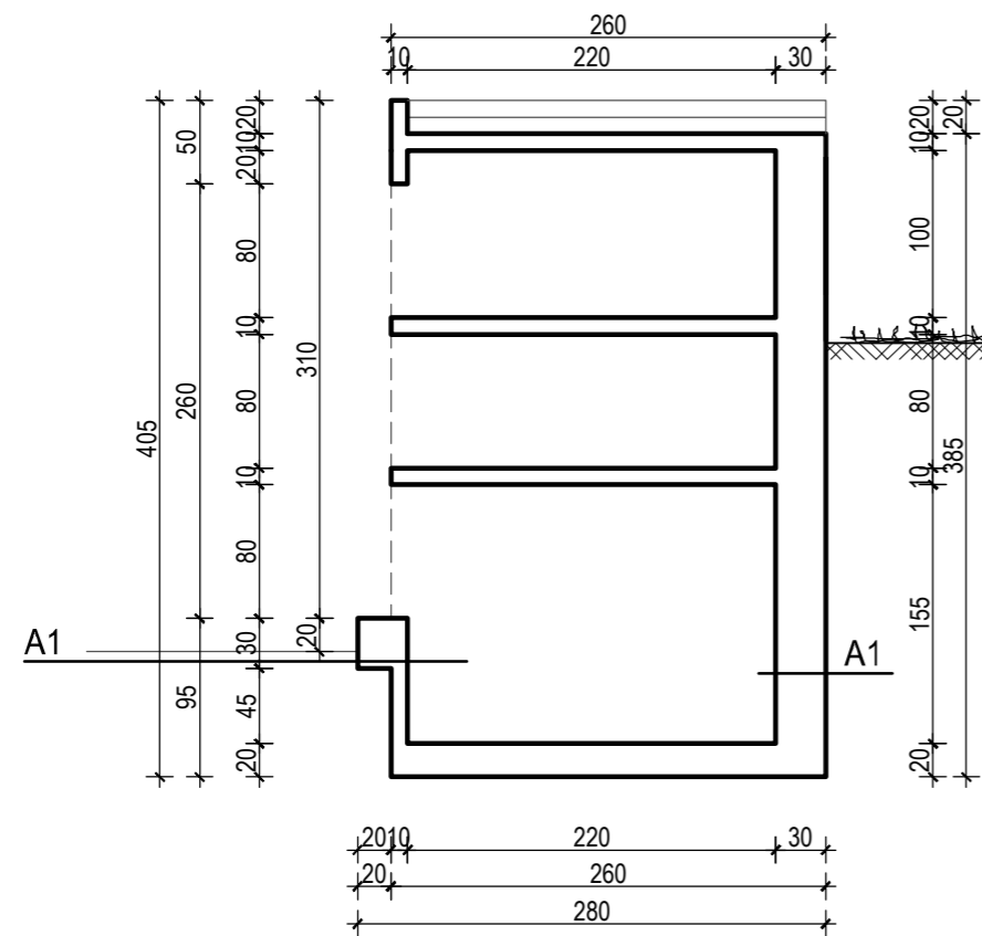
PRESJEK B1-B1
